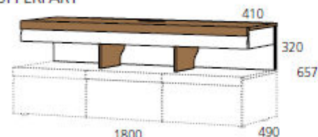
PZ-TVN6 (1 KLOPNA VRATA / POKLOPNA VRATA / FLAP DOOR)
